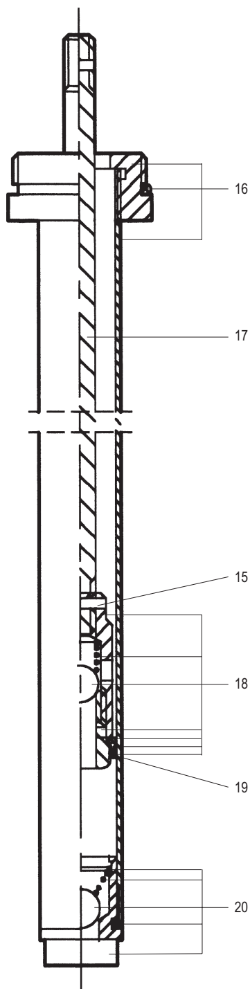
Pump tube/pumprör 15780-81
