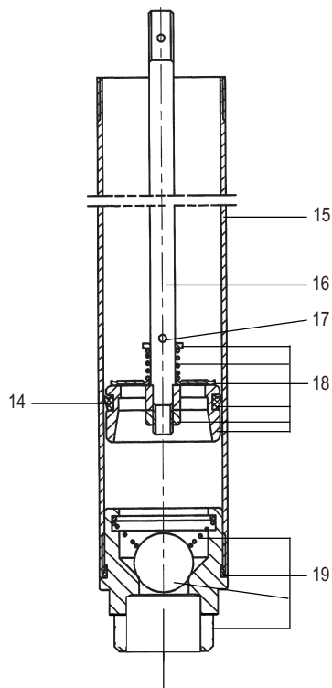
Pump tube/pumprör A11740-10
