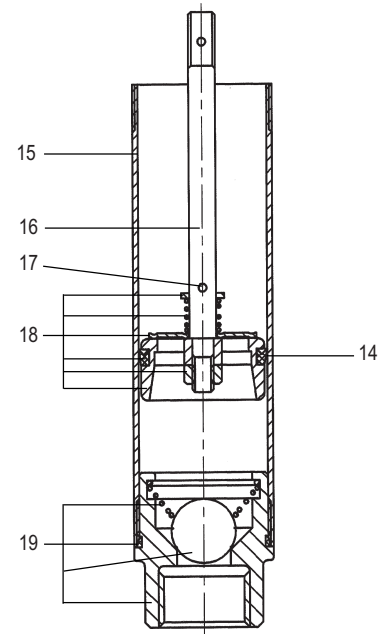
Pump tube/pumprör A11741-10
