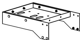
EXTENDER FOR TWO EXTRA HOSE REELS / FÖRLÄNGNING FÖR TVÅ EXTRA SLANGUPPRULLARE
