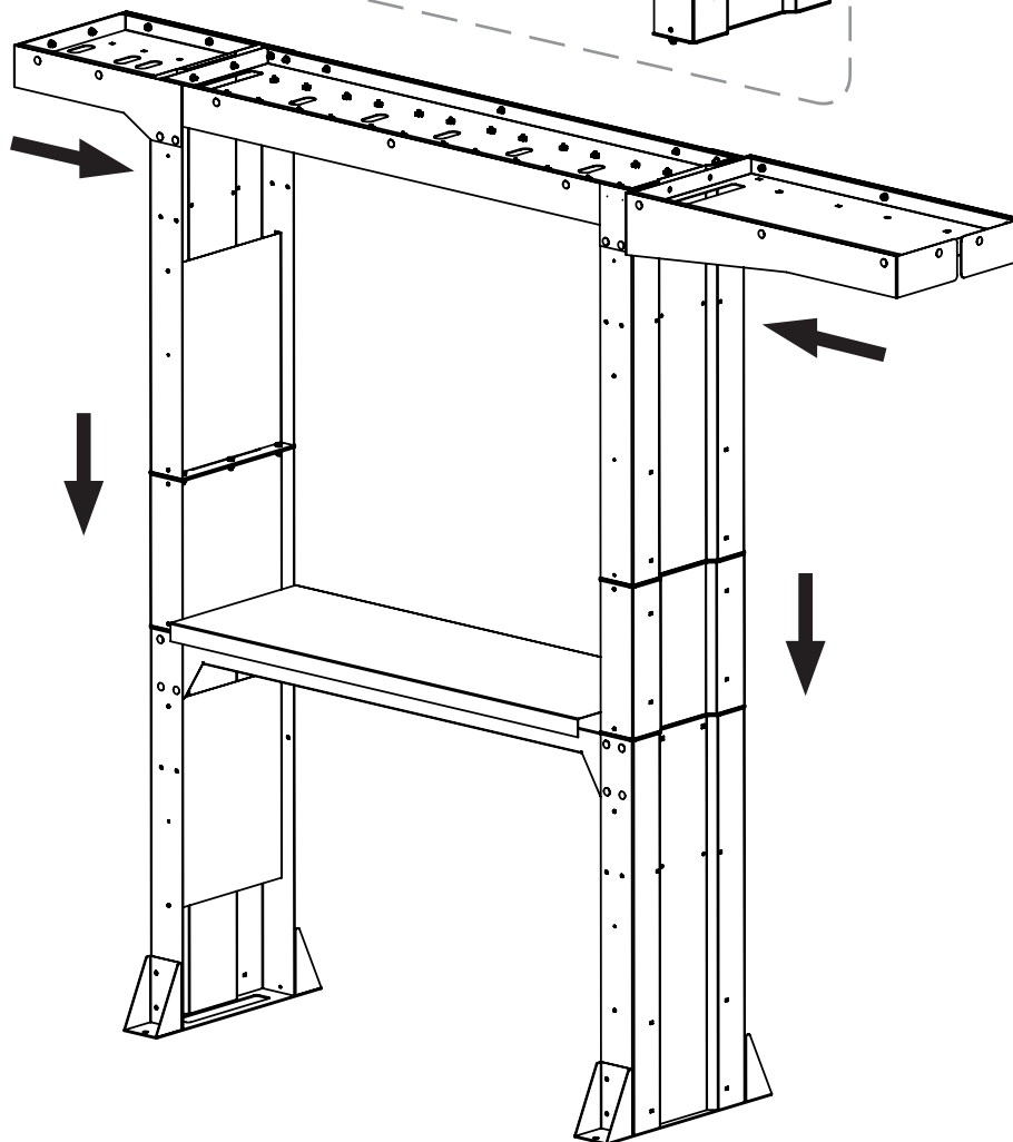
HEIGHT EXTENDER / FÖRLÄNGNING
